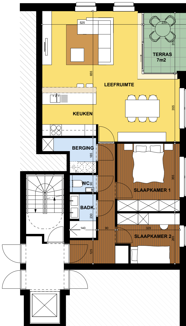
APPARTEMENT 3.4 niveau 3 - 80m 2 excl. terras
